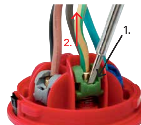
Demontage: Klem met schroevendraaier openen, kabel eruit trekken
